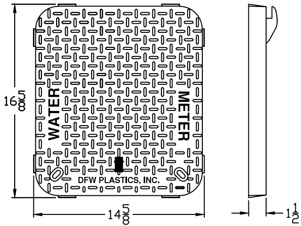
DFW39C-1-LID
