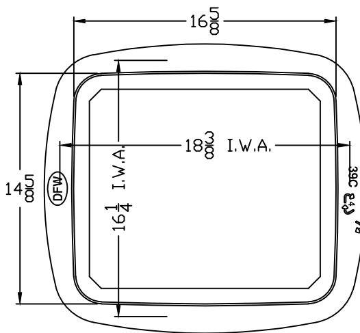
DFW39C-1-LID
